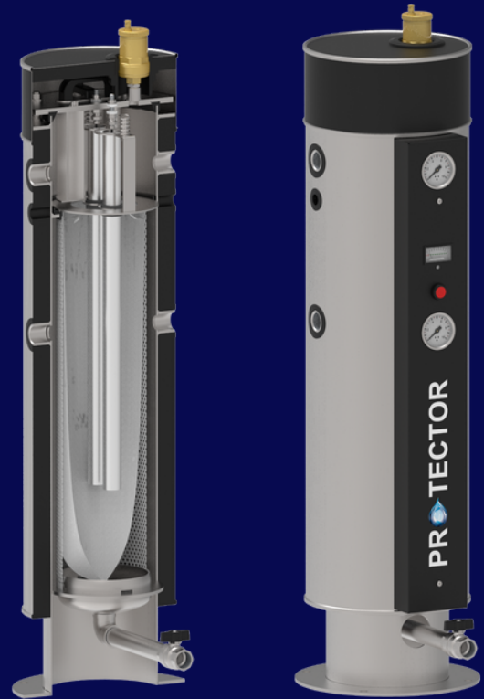
Snitt som viser øvre kammer med magneter før man kommer ned i selve partikkel filter og anode kammer
